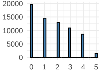
ed_sde
