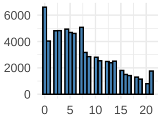
anx_score
