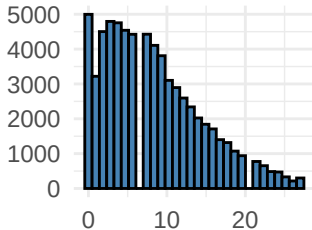
deprawsc
